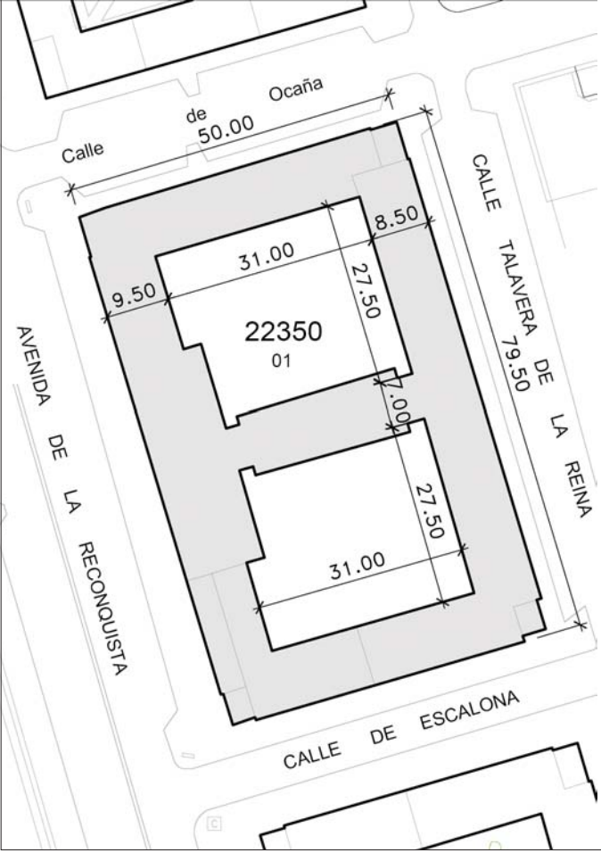
DESCRIPCIÓN GRÁFICA 1:1.000
